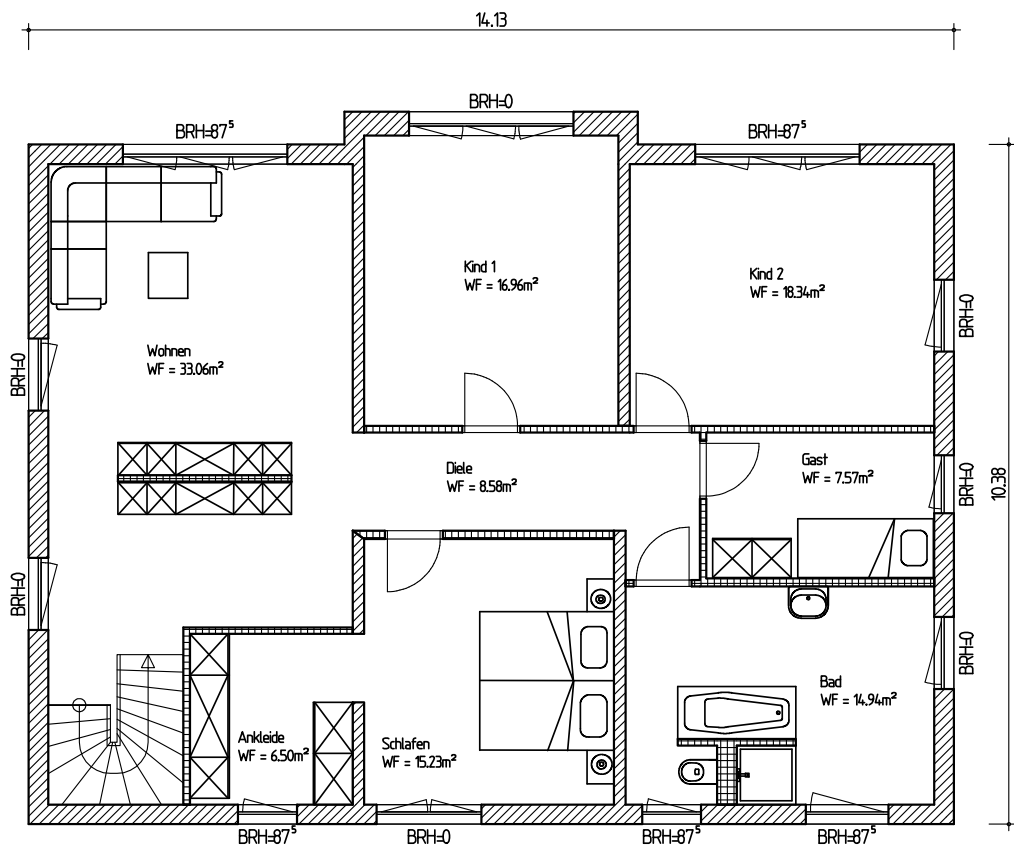
Obergeschoss
